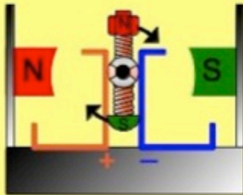
1. elettromagneti attivi
