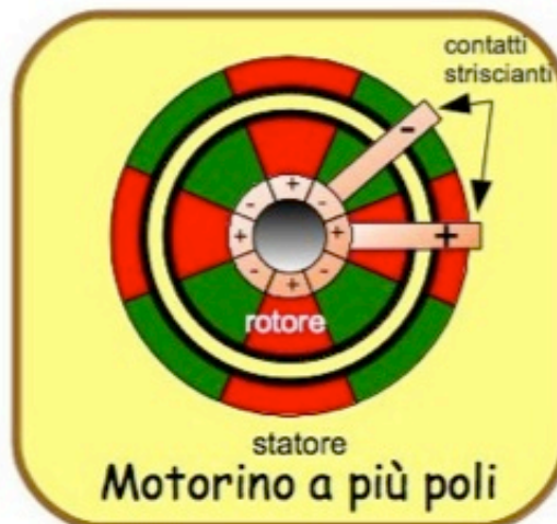
Contatti aperti
