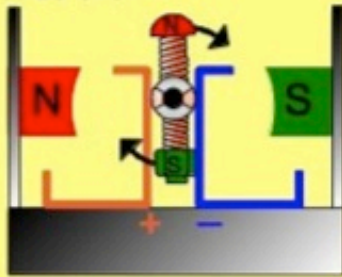
3. elettromagneti attivi e invertiti
